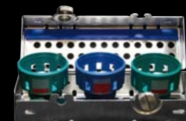
Piezo spets Guardian momentnyckelkassett – IMIQ38. (Ej DIN format.)
